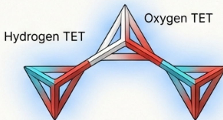
H 2 O (Water)
