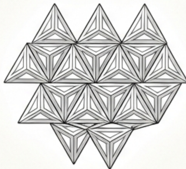
C (Diamond)
